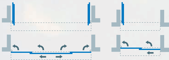
Четырехстворчатая FBO 2 подвижные-распашные 2 распашные
